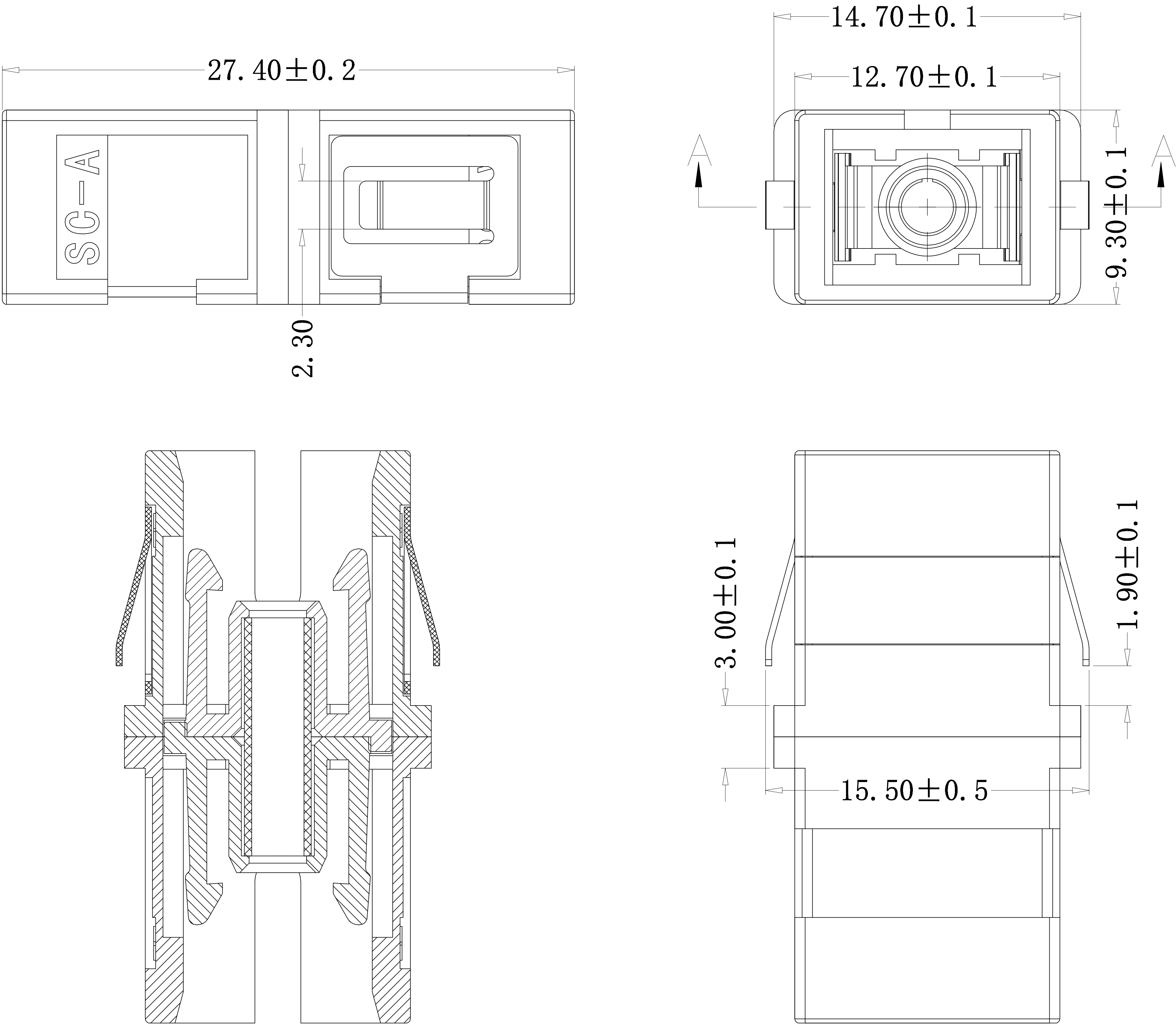
SECTION A-A
